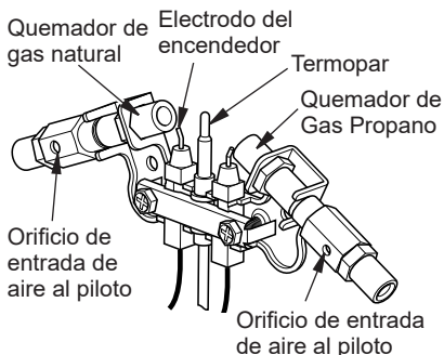
Figura 26 - Orificio de entrada de aire al piloto
