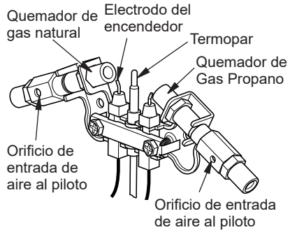
Figura 21 - Conjunto de piloto
