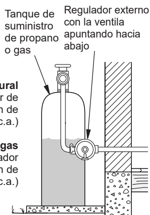
Figura 16 - Regulador externo con la ventila apuntando hacia abajo (sólo propano o gas)
