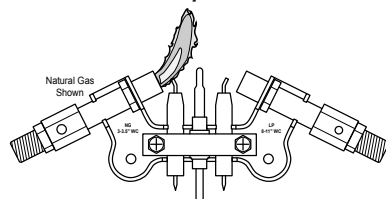
Figura 23 - Patrón incorrecto de la llama del piloto
