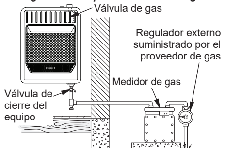
Figura 19 - Suministro de gas natural
