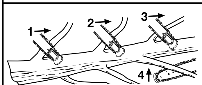
COUPER LES BRANCHES UNE À UNE ET LAISSER CELLES SOUTENANT LE TRONC JUSQU'À CE QUE CELUI-CI SOIT DÉBITÉ.
