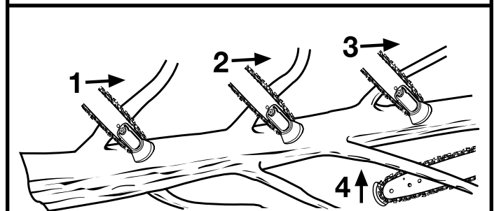
CORTE UNA RAMA A LA VEZ Y DEJE RAMAS DE SOPORTE BAJO EL ÁRBOL HASTA QUE ESTÉ CORTADO EL TRONCO
