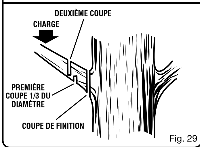
COUPER LES BRANCHES UNE À UNE ET LAISSER CELLES SOUTENANT LE TRONC JUSQU'À CE QUE CELUI-CI SOIT DÉBITÉ.
