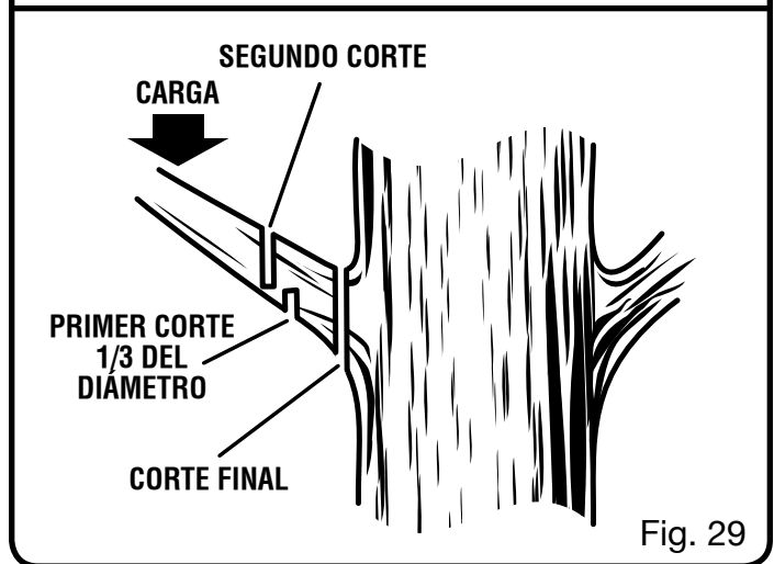
CORTE UNA RAMA A LA VEZ Y DEJE RAMAS DE SOPORTE BAJO EL ÁRBOL HASTA QUE ESTÉ CORTADO EL TRONCO
