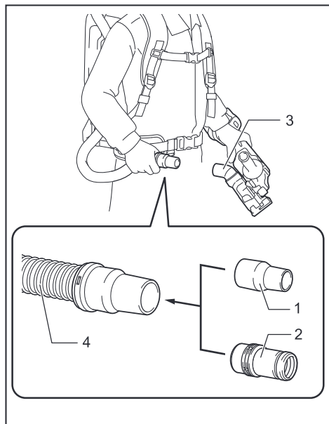
► 1. Junta 2. Boca delantera 3. Salida de extracción 4. Manguera
