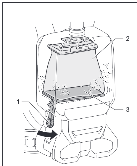
► 1. Palanca 2. Bolsa del filtro/bolsa recolectora de polvo 3. Tablero
