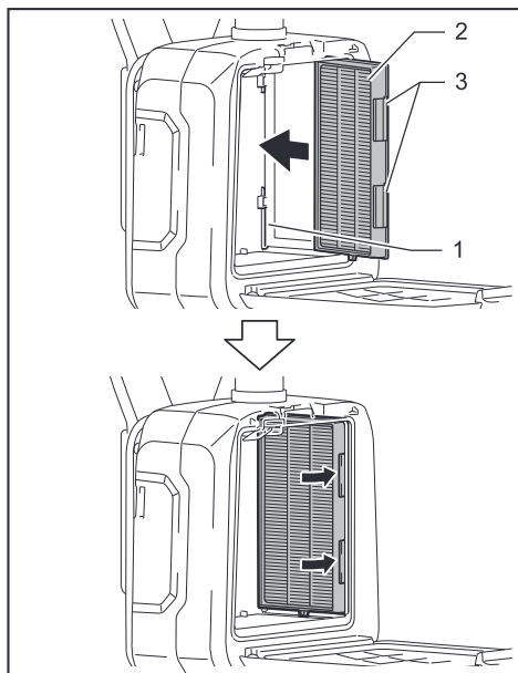
► 1. Ranura 2. Filtro HEPA 3. Gancho
