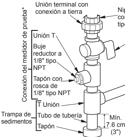
Figura 11 - Conexión de gas
