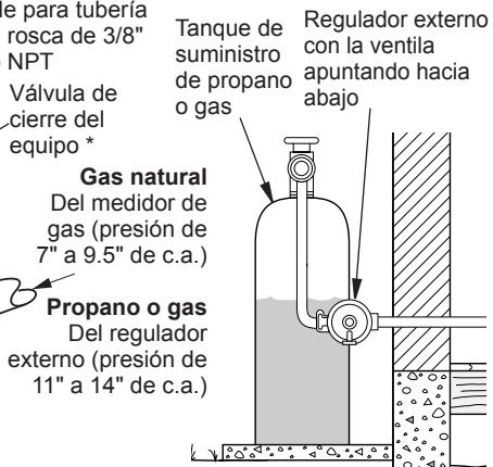
Figura 12 - Regulador externo con la ventila apuntando hacia abajo (sólo propano y gas)
