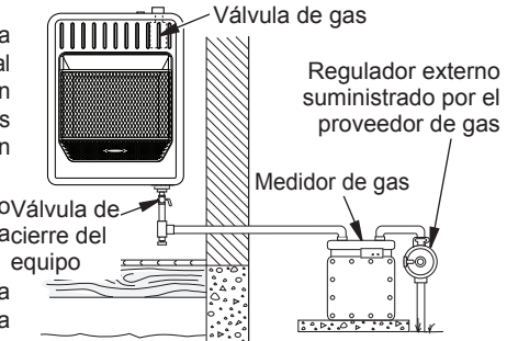
Figura 14 - Suministro de gas natural
