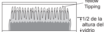
Figura 23 - Patrón incorrecto de la llama del quemador
