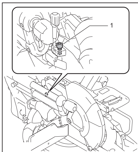
► 1. Adjusting bolt
