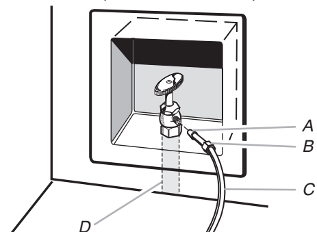
C. Canalisation en cuivre (jusqu'au réfrigérateur) D. Canalisation d'alimentation en eau du domicile (1/2 po minimum)
