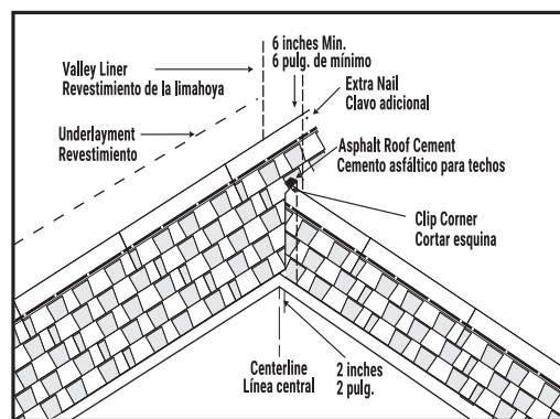
Fig. 6 Closed-Cut Valley Construction Construcción de limahoya con corte cerrado
