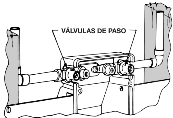
Ilustración de la caja ranurada con válvulas de paso instaladas.
