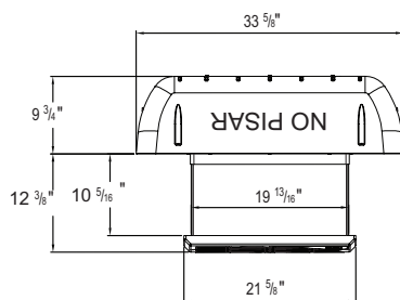
VISTA SUPERIOR
