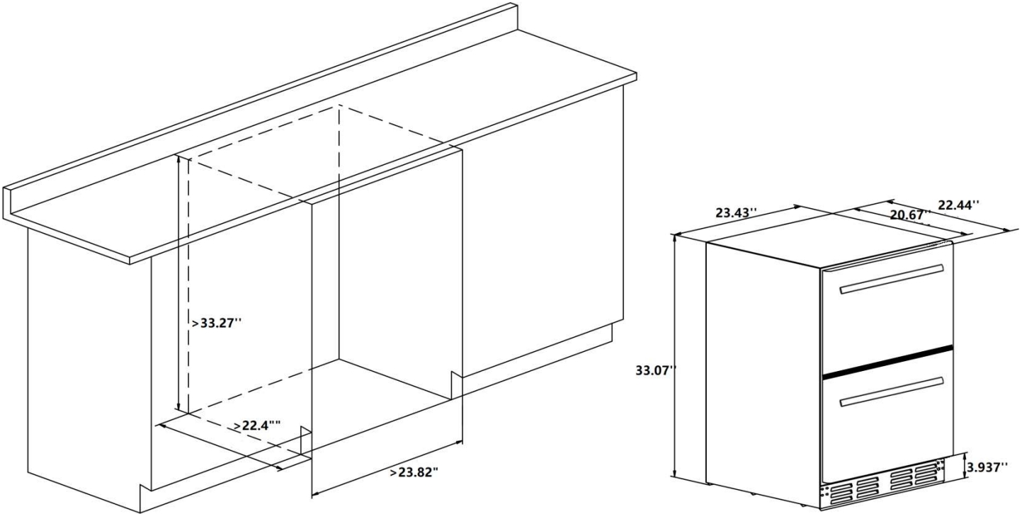
KRC-150DF
