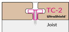
TC-2 (CEC Clip)
