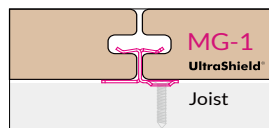
MG-1 (CEC Clip)
