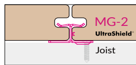
MG-2 (Locking Clip)
