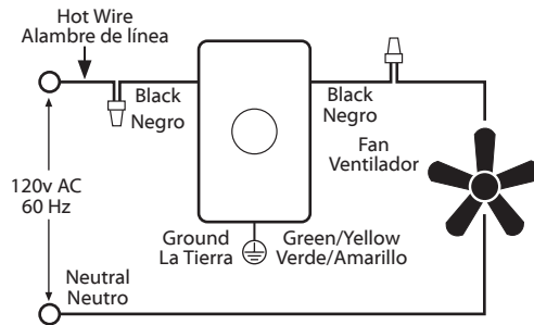
Wiring Diagram Diagrama de cableado
