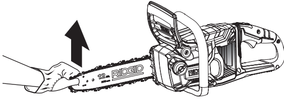
Fig. 32 LIFT THE TIP OF THE GUIDE BAR UP TO CHECK FOR SAG RELEVER L'EXTRÉMITÉ DU GUIDE POUR VÉRIFIER LE MOU LEVANTE LA PUNTA DE LA BARRA GUÍA PARA REVISAR LA HOLGURA DE LA CADENA
