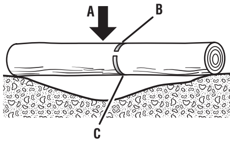
LOG SUPPORTED AT BOTH ENDS: BILLE SOUTENUE AUX DEUX EXTRÉMITÉS : TRONCO APOYADO POR AMBOS EXTREMOS :
