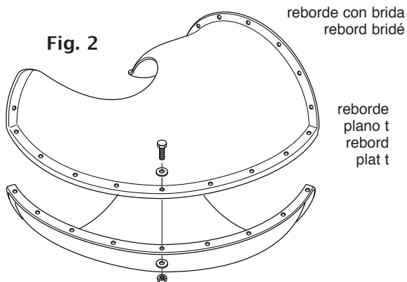
Sección de Salida - 13 pernos Section de sortie - 13 boulons
