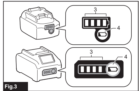
► 3. Lámparas indicadoras 4. Botón de verificación
