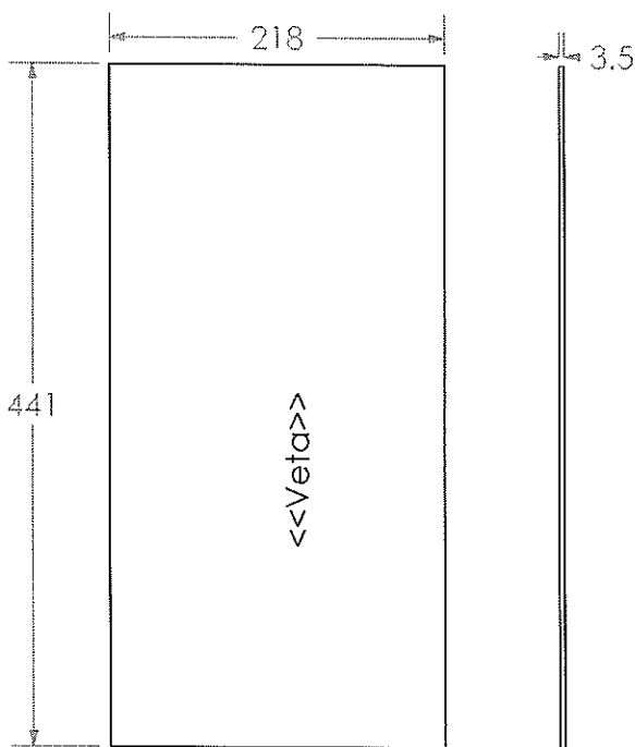
Respaldo Vista Superior
