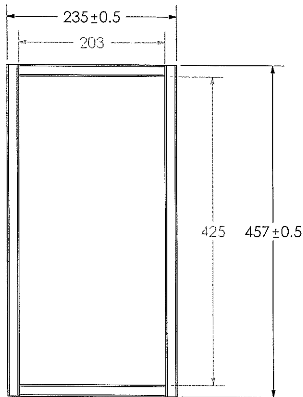
Ensamble de Cajon Vista Superior
