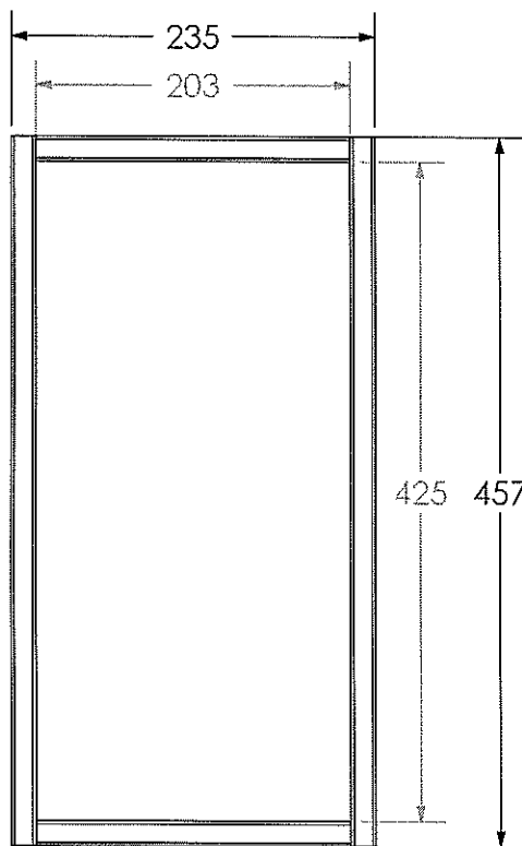
Ensamble de Cajon Vista Superior
