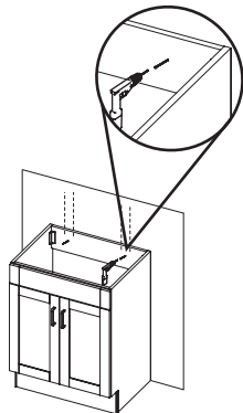
back top rail rail arrière supérieur soporte superior trasero
