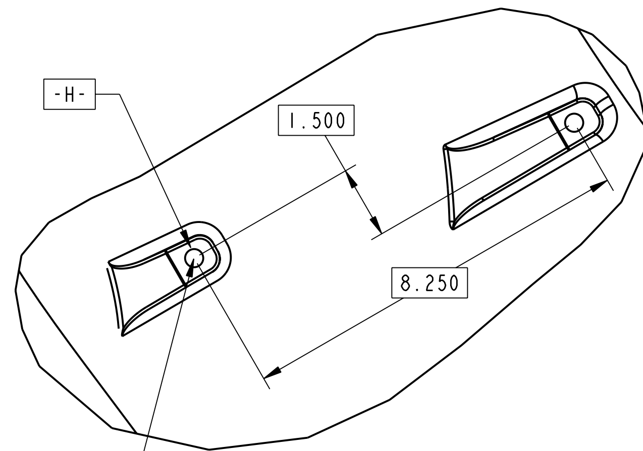
LUG DETAIL SCALE 0.500
