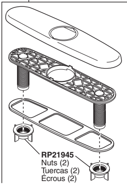
RP47274▲ Optional Escutcheon, Plate, Nuts and Gasket Chapa Opcional, Placa, Tuercas y Empaque Plaque de finition facultative, plaque, écrous et joint
