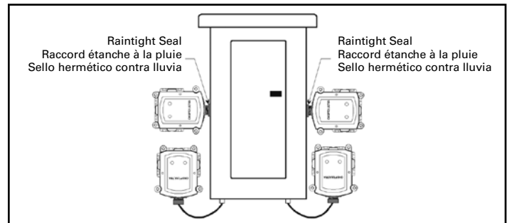
Figure 5. Outdoor Installation (2)/Installation à l'extérieur (2)/Instalación exterior
