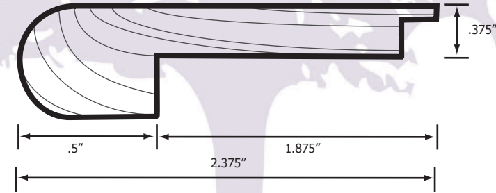
Flushmount Stairnose- EGD 1/2"
