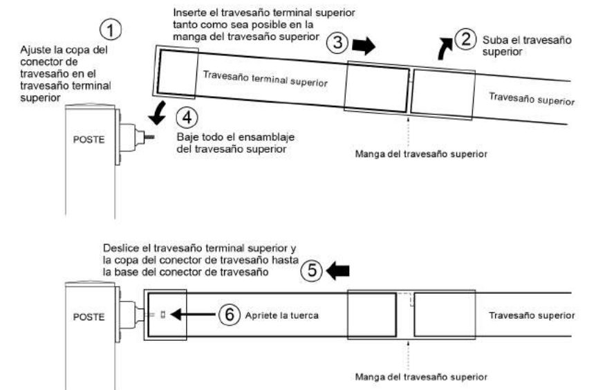
Fig. 11 Inserción del travesaño terminal superior
