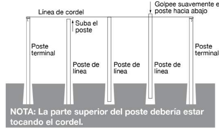
Fig. 6 Nivele los postes para que estén a la misma altura respecto a la superficie del terreno.
