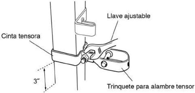
Fig. 12 Instalación de la cinta tensora
