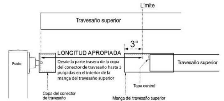
Fig. 11 Inserción del travesaño terminal superior
