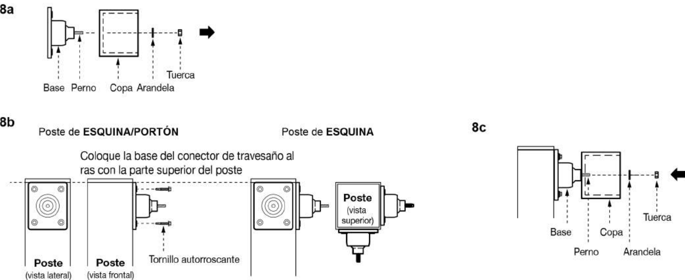
Fig. 8 Ensamblaje de conector de travesaño
