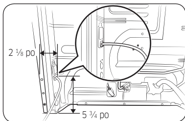
Emplacement du cordon d'alimentation
