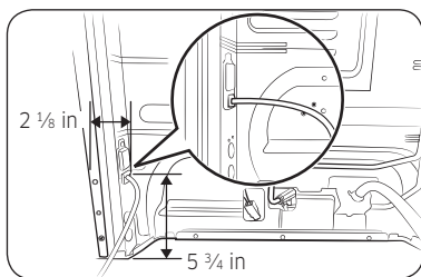
Ubicación del cable de alimentación
