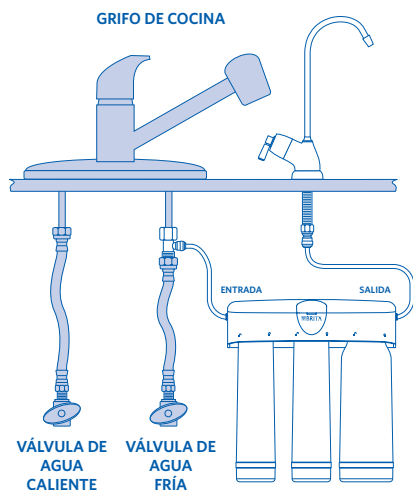
INSTALACIÓN CON TUBERÍA FLEXIBLE
