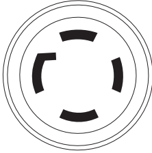
Figura 2-7. Receptáculo de 120/240 V CA, 30 A NEMA L14-30R
