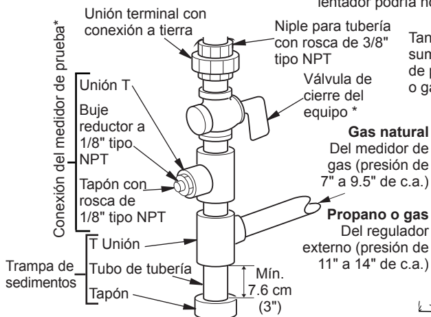
Figura 11 - Conexión de gas
