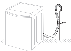
Raccordement du tuyau de vidange
