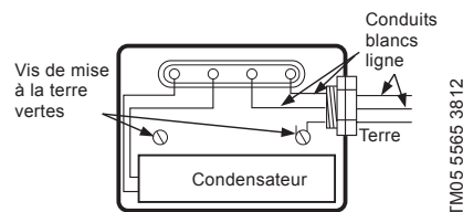
Fig. 3 Schéma de câblage pour toutes les pompes 115 V et 230 V à vitesse unique.
