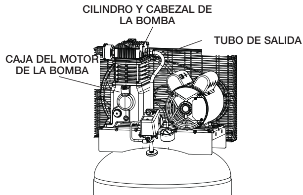
Fig. 1 Superficies calientes
